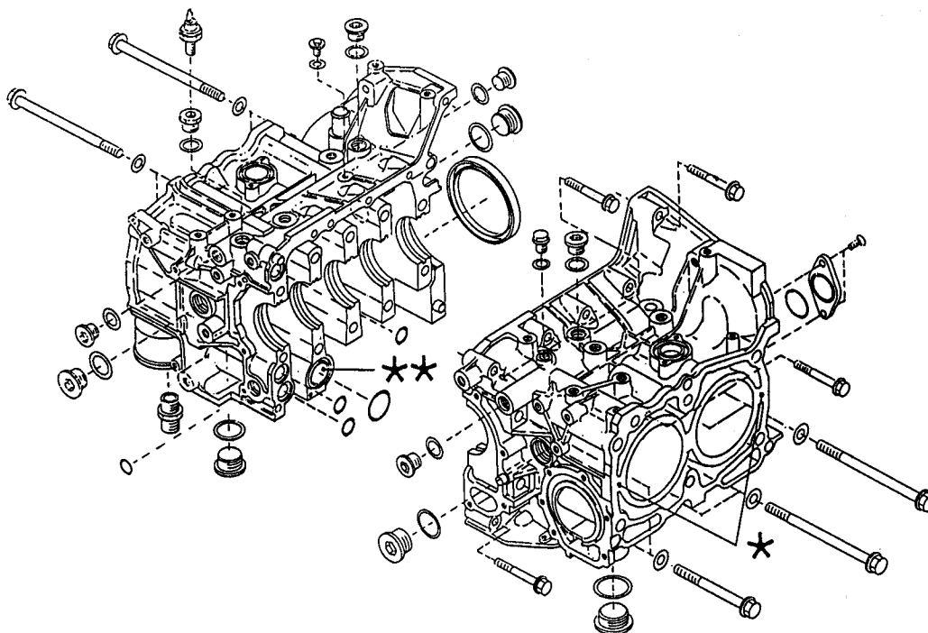
Fig. 6 Crankcase
