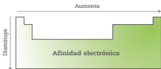
Figura 2.48 Tendencia de la afinidad electrónica.
