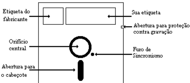
Um disco flexível de 5¼ polegadas
