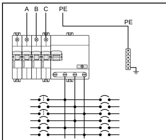
Alimentação 3 Fases
