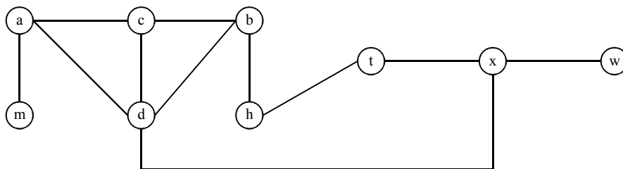
Grafo conexo
