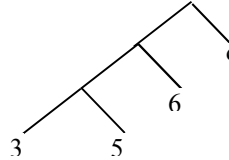
Árbol_2 P(\text{Árbol}_2) = 45
