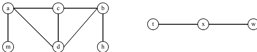
Grafo no conexo
