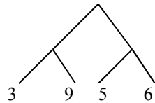
Árbol_1 P(\text{Árbol}_1) = 46
