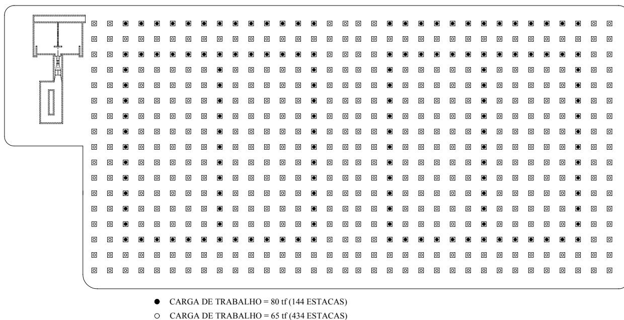
Figura 2 – Tanques de Decantação - Locação de Estacas (578 Estacas Pré-Moldadas)
