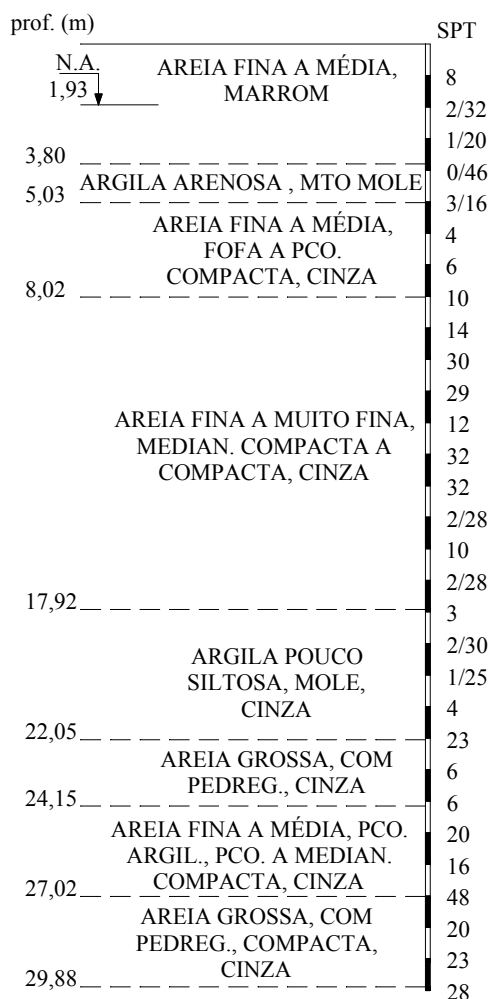
Figura 1 – Perfil Geológico Geotécnico Típico do Local de Implantação da Obra
