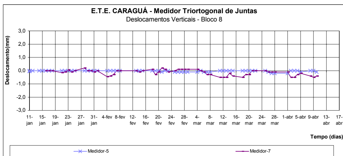
Figura 5 – Gráficos com Leituras do Medidores Triortogonais (Deslocamentos Verticais - Bloco 8)
