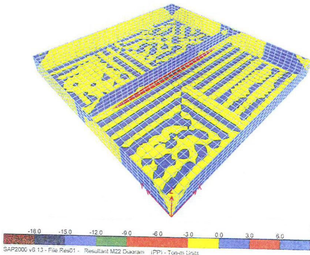
Figura 3 – Diagramas de Esforços Solicitantes (SAP 2000 – Momentos Fletores), considerando os recalques previstos.
