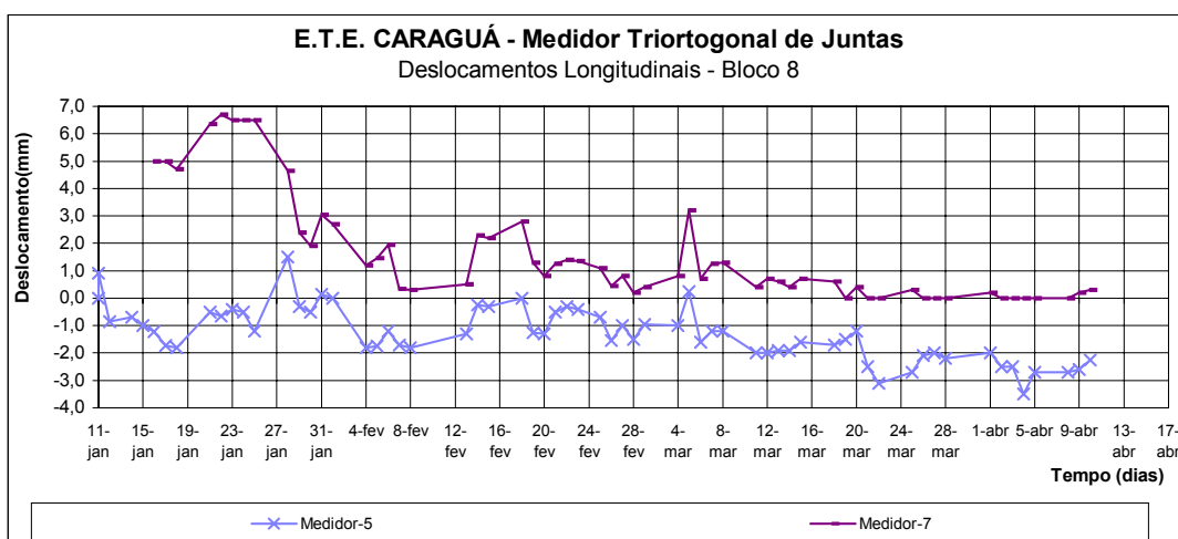
Figura 7 – Gráficos com Leituras do Medidores Triortogonais (Deslocamentos Transversais - Bloco 8)
