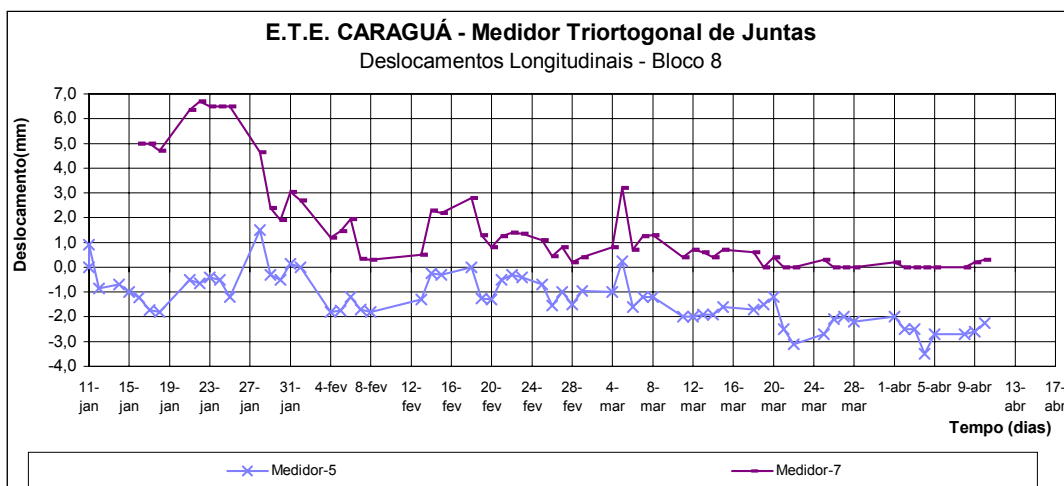
Figura 6 – Gráficos com Leituras do Medidores Triortogonais (Deslocamentos Longitudinais - Bloco 8)
