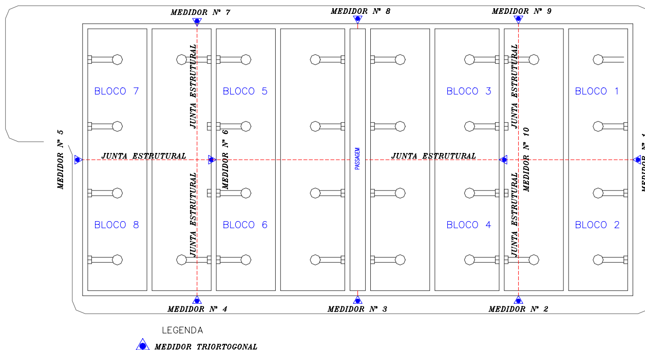
Figura 4 – Planta de Locação dos Medidores Triortogonais
