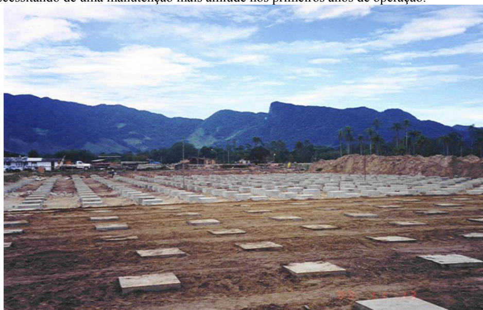
Foto 1 – Vista dos Capitéis sobre Estacas de Concreto Pré-moldadas, com o Reaterro em Execução.
