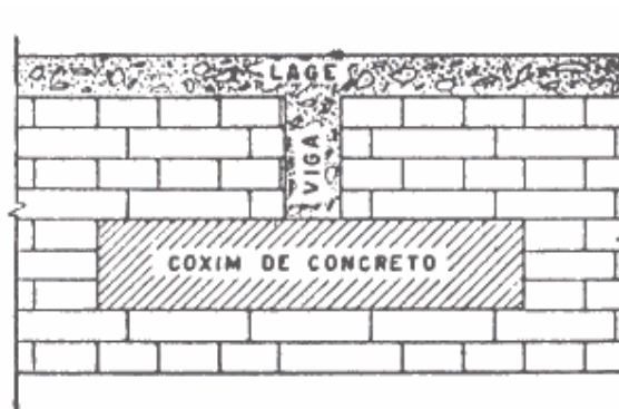
Figura 32. Cxim de concreto.
