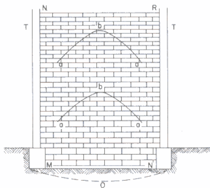
Figura 39. Fissuras parabólicas.
