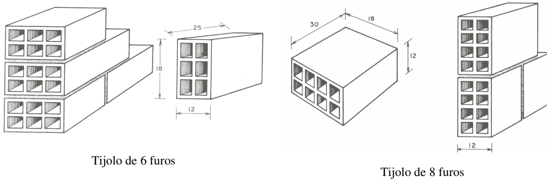
Figura 4. Tijolos furados.
