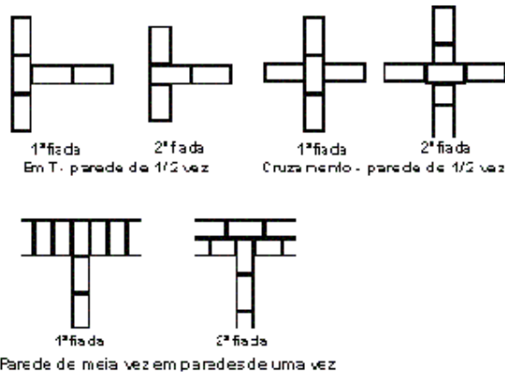
Figura 27. Amarração em cruzamento.
