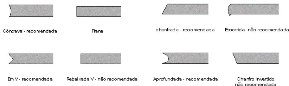
Figura 28. Tipos de juntas.
