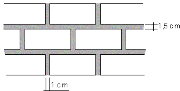
Figura 12. Juntas desencontradas.
