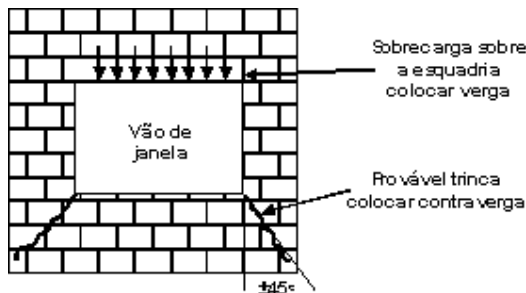
Figura 17. Verga e contraverga em vão de janela.
