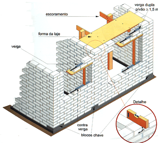
Figura 37. Colocação de vergas e contravergas.
