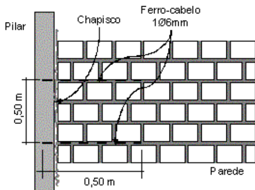
Figura 33. Ligação da parede com pilar.
