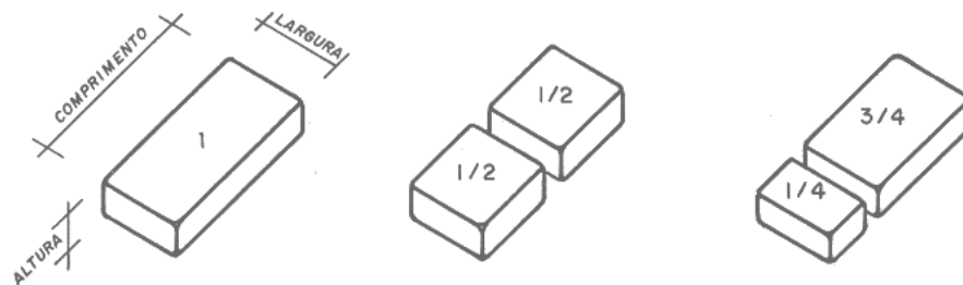
Figura 3. Formas de corte do tijolo.
