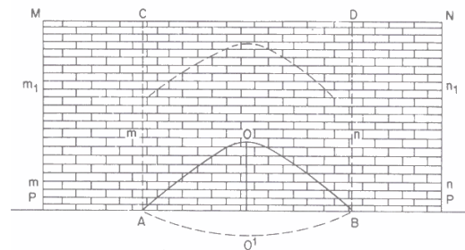
Figura 40. Fissuras em forma de parábola alongada.
