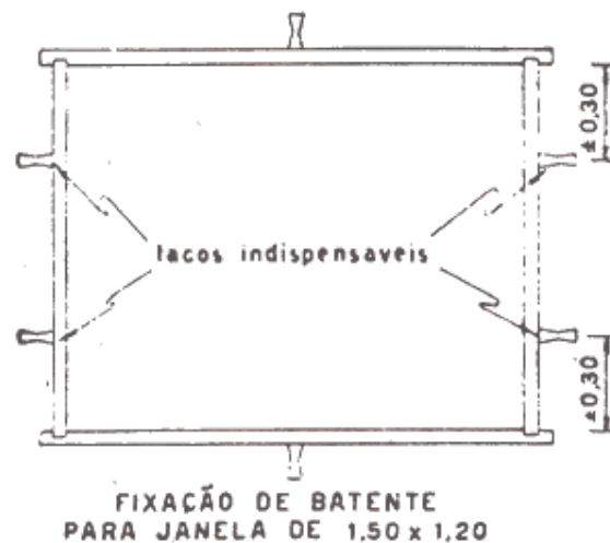
Figura 20. Tacos para fixação de batentes de janelas.
