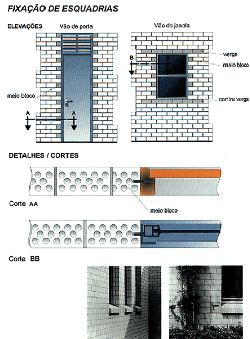
Figura 38. Fixação das esquadrias.
