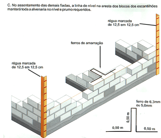
Figura 36. Assentamento das fiadas subsequentes.
