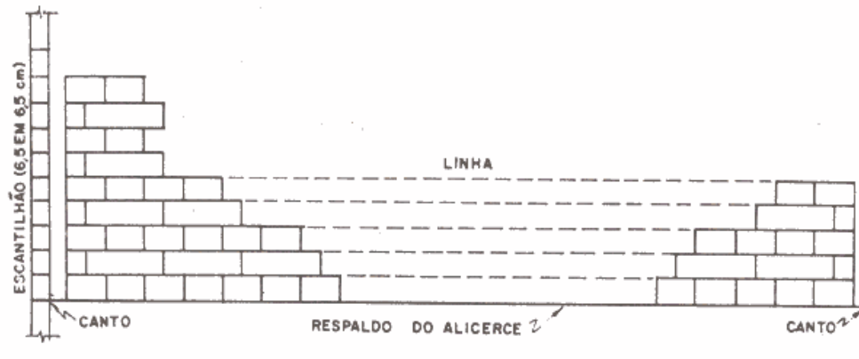
Figura 15. Execução de parede de alvenaria.
