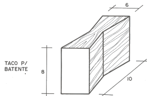
Figura 19. Dimensões do taco de madeira para batente.
