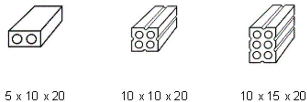
Figura 5. Tijolos furados – tipo 1.
