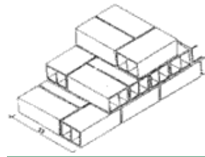
Figura 10. Alvenaria de um tijolo e meio.
