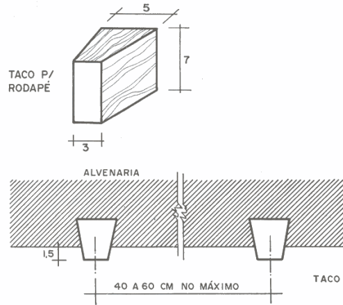
Figura 22. Dimensões e espaçamento de tacos de rodapé.
