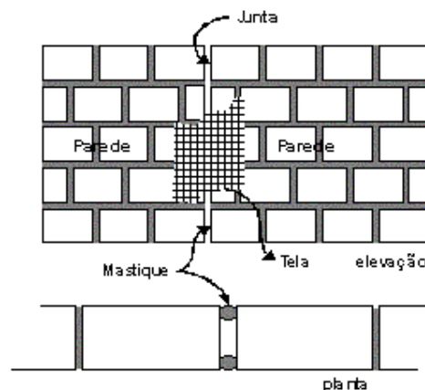
Figura 34. Ligação de parede com parede, sem amarração.
