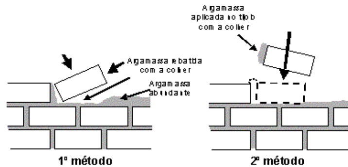
Figura 13. Métodos de espalhamento da argamassa.
