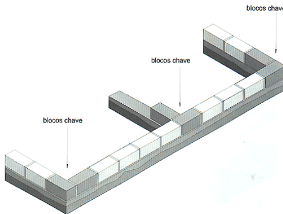
Figura 35. Execução da primeira fiada.
