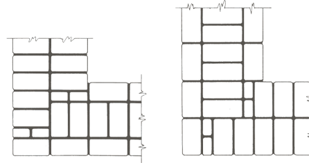
Figura 26. Alvenaria de dois tijolos.
