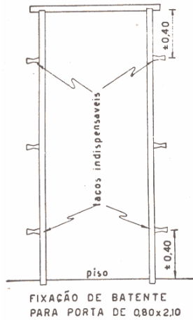
Figura 21. Tacos para fixação de batentes de portas.
