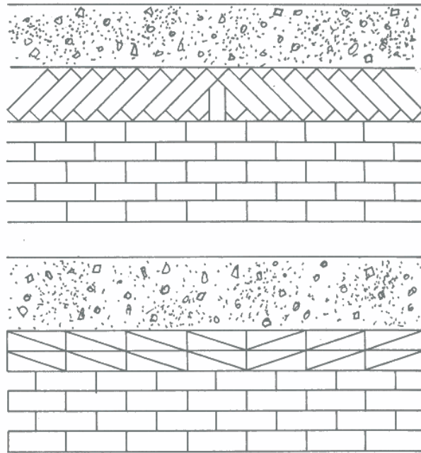
Figura 29. Encunhamento com tijolos maciços.
