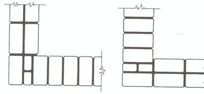
Figura 24. Alvenaria de um tijolo.
