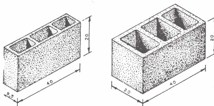
Figura 6. Bloco de concreto.
