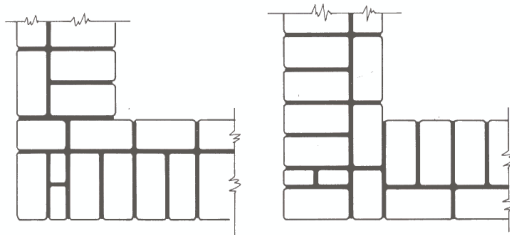
Figura 25. Alvenaria de um tijolo e meio.
