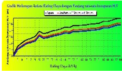
Grafik 6. Hubungan Rating daya – panjang rata-rata kumparan H.V dengan variasi core section
