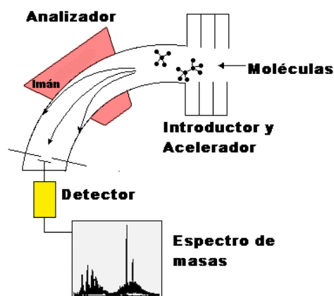
Figura 1. Esquema de los equipos de espectrometría de masas. La introducción e ionización de la muestra se esquematizan como cámaras separadas.
