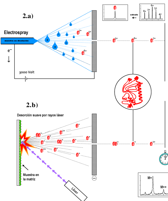
Figura 2. a) Esquema del sistema de electrospray. b) Sinopsis del método de ionización suave por rayos láser. En ambos casos la relación m/z es determinada por tiempo de vuelo y se obtienen iones policargados.
