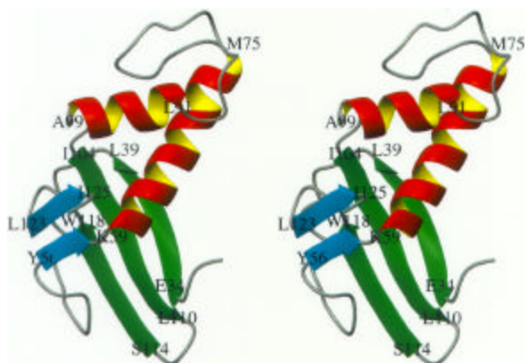
Figura 4. Representación estereográfica de la estructura de la proteína h-RPABC subunidad de la RNA polimerasa humana (Nature Structural Biology, 6 (1999) 1039-1042).
