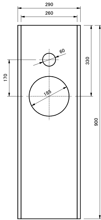
TR130d Assembly
