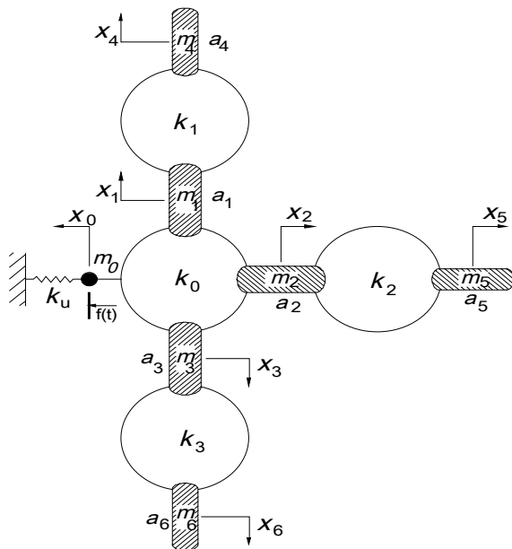
Fig.1 振動モデル
