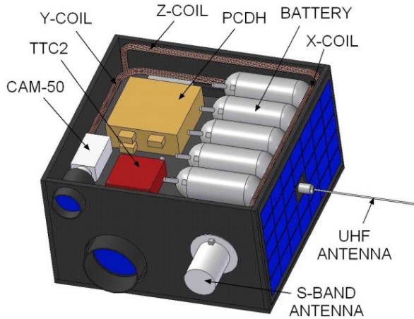
Gambar-1(a) Kompartemen Atas.
