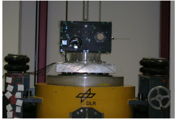
Gambar 9. Pengujian pada axis Y
