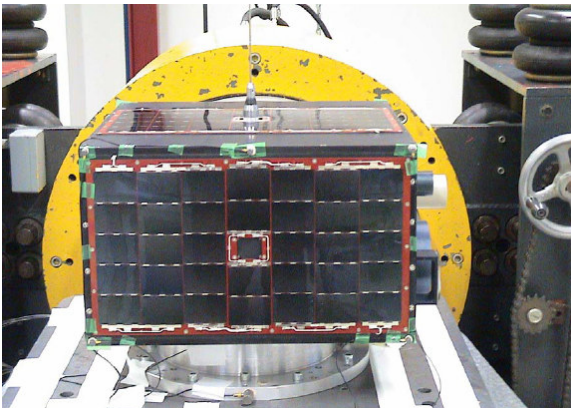
Gambar 8. Pengujian pada axis X
