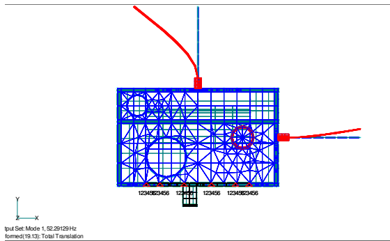
Gambar 4. Modus resonansi pada 52.29 Hz
