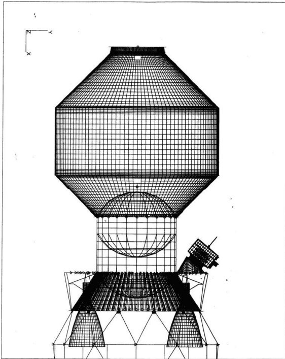
Gambar 7. Model LAPAN-TUBSAT pada analisa beban payload PSLV C7
