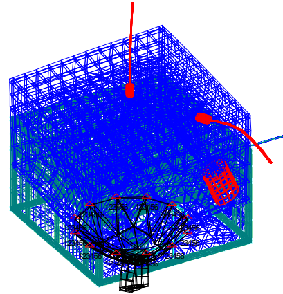
Gambar 6. Modus resonansi pada 151.47 Hz
