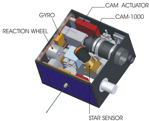
Gambar-1(b) : Kompartemen Bawah
