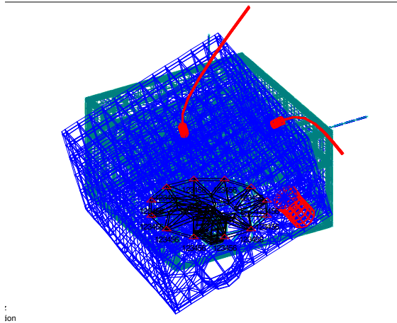
Gambar 5. Modus resonansi pada 104.09 Hz
