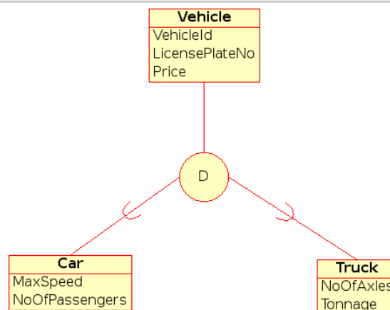
Representación visual de una especialización de separación en un diagrama EER
