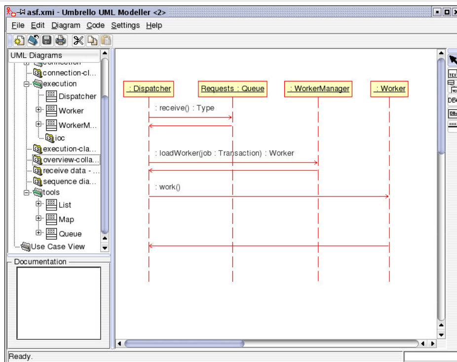
Umbrello UML Modeller mostrando un diagrama de secuencia
