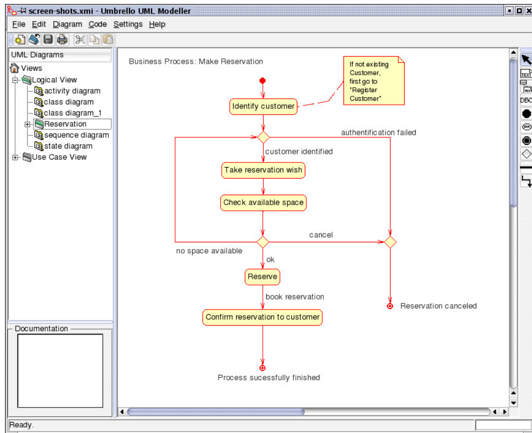
Umbrello UML Modeller mostrando un diagrama de actividad
