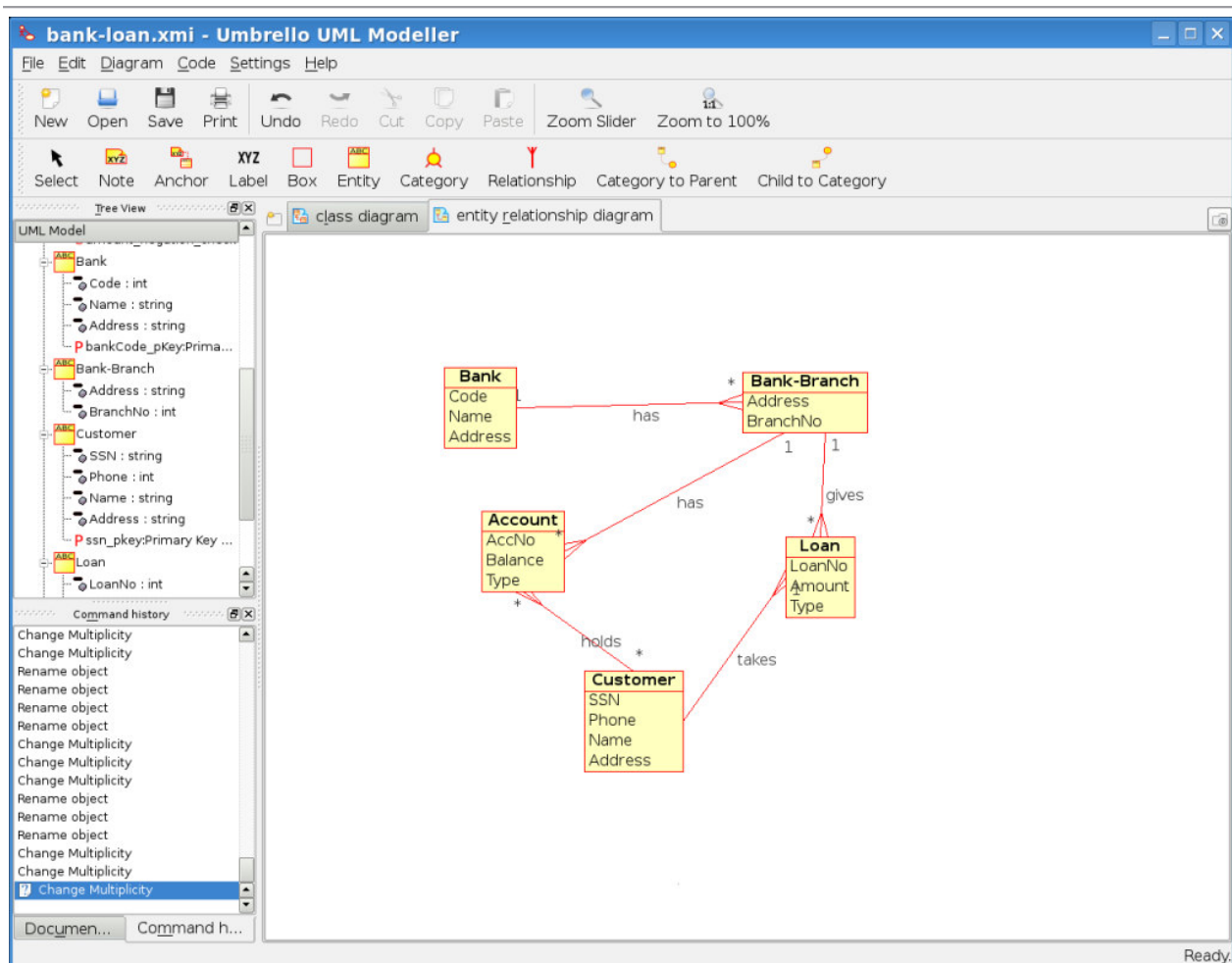
Umbrello mostrando un diagrama de relaciones de entidad
