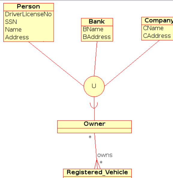
Representación visual de una categoría en un diagrama EER
