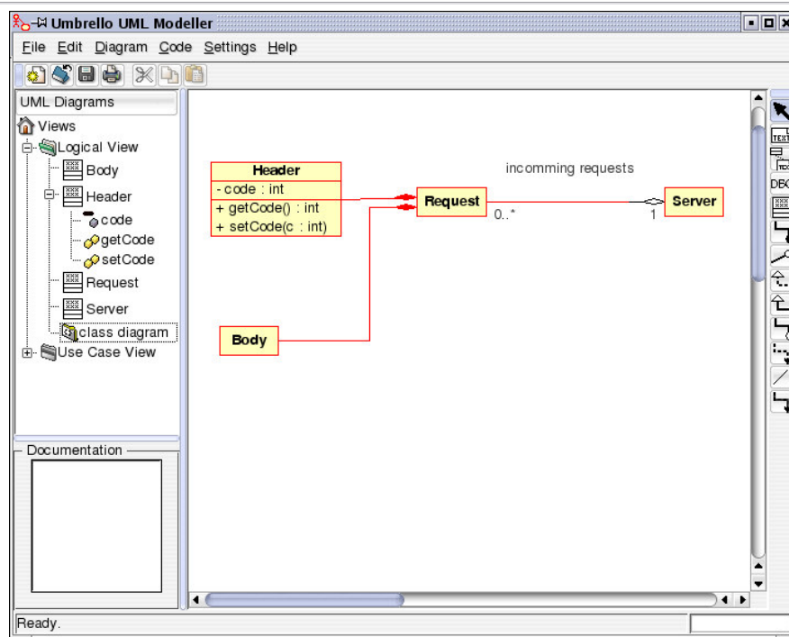
Umbrello UML Modeller mostrando un diagrama de clases
