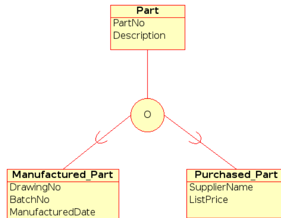
Representación visual de la especialización de solapamiento en un diagrama EER
