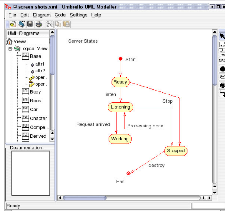
Umbrello UML Modeller mostrando un diagrama de estado
