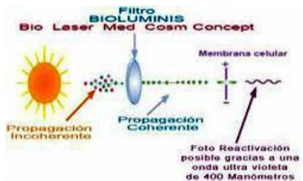
Figura 5: Coherencia de los biofotones según ref. [1] Aunque no hay un consenso general respecto a estos
