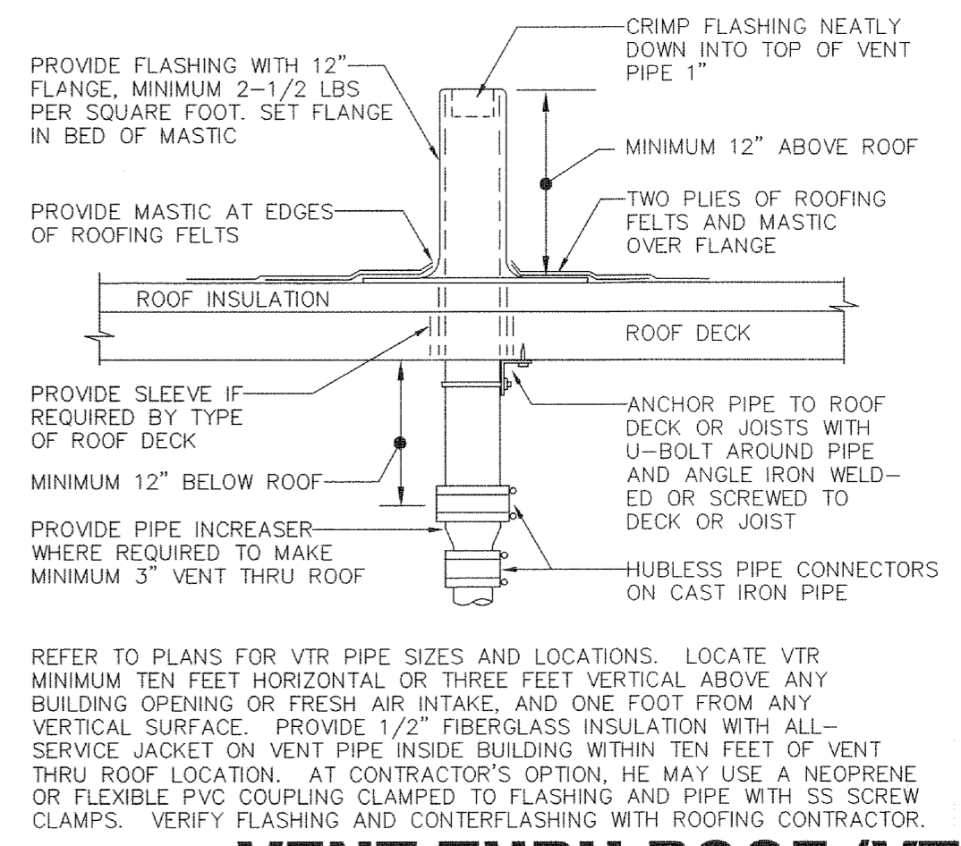
5 VENT THRU ROOF (VTR) SCALE: NO SCALE
