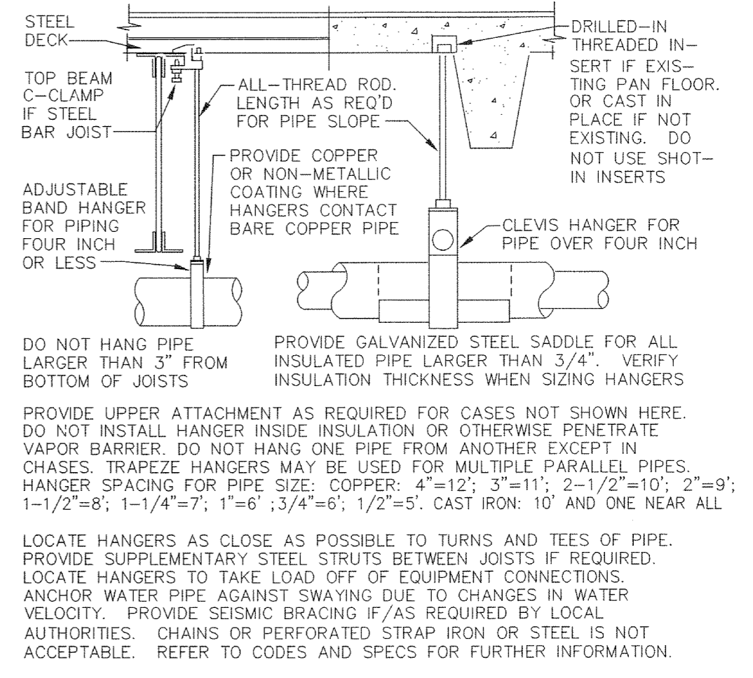
2 PIPE HANGER SCALE: NO SCALE
