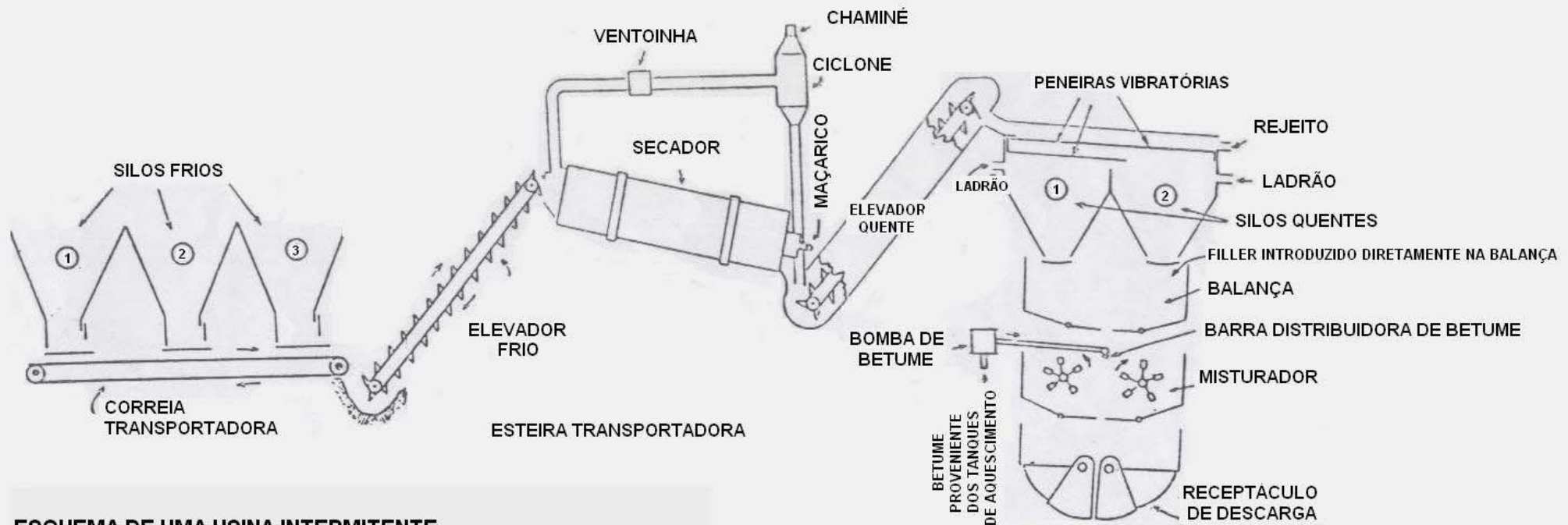
ESQUEMA DE UMA USINA INTERMITENTE
