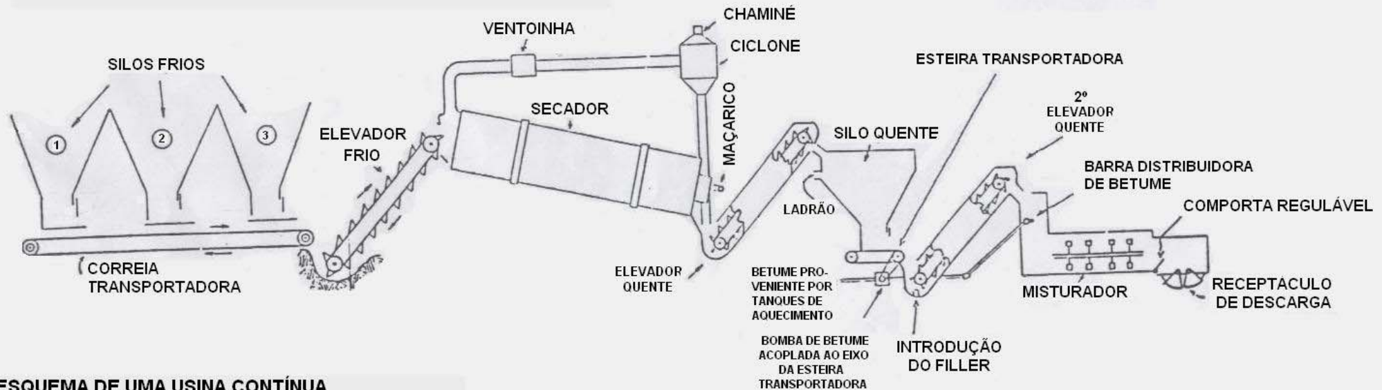
ESQUEMA DE UMA USINA CONTÍNUA
