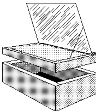
Figura G.6 - Forno solar pronto. Pode-se ver a tampa removível, tendo o filme plástico na parte central com a aba coberta com papel alumínio, levantada pelo arame e o corpo do forno onde se vê o fundo preto e as laterais espessas, com ar dentro, formadas pelas duas caixas. Redesenhado a partir de desenho de Mark Aalfs [9] em http://solarcooking.org/sbcdes.htm .
