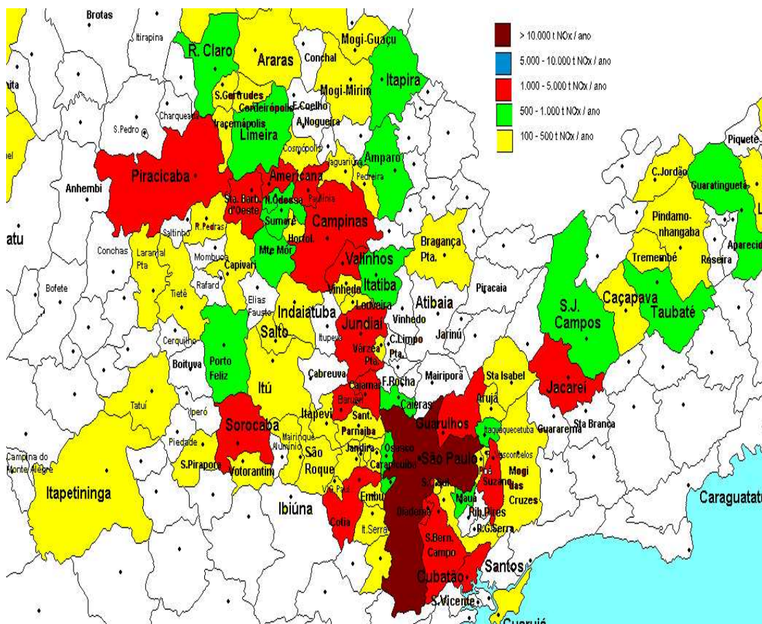
Figura 4.14. Emissões de NO_x por município, cenário Alto, 2000.
