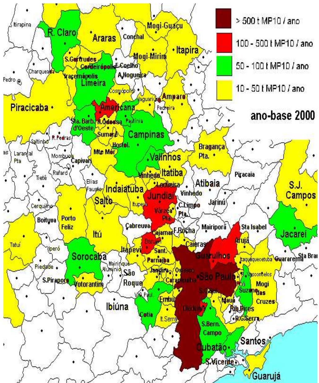
Figura 4.23. Emissões de MP_{10} nos eixos da Capital, cenário Alto, 2000.
