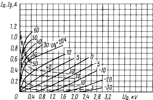
Усредненные анодные и сеточно-анодные характеристики: U_i = 12,6 \text{ В} — анодные; - - - сеточно-анодные Averaged Anode and Grid-Anode Characteristic Curves: U_i = 12.6 \text{ V} — anode; - - - grid-anode
