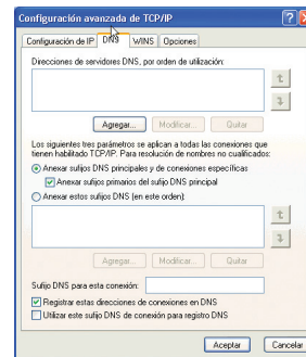
Figuras 7.10 Panel de control avanzada de TCP/IP
