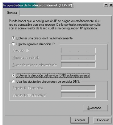
Figura 6.21 Propiedades de Protocolo Internet (TCP/IP)
