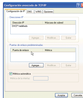
Figuras 7.10 Panel de control avanzada de TCP/IP
