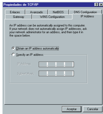
Figura 4.17 (a) TCP/IP (Dirección IP)
