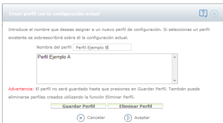
-Figura 5.13-
