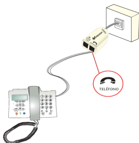
Figura 3.1 Cableado en el microfiltro doble salida
