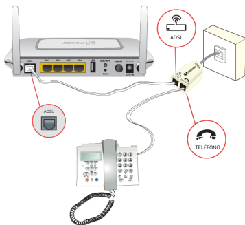
Figura 3.3 Conexión del Home Station ADSL a la roseta
