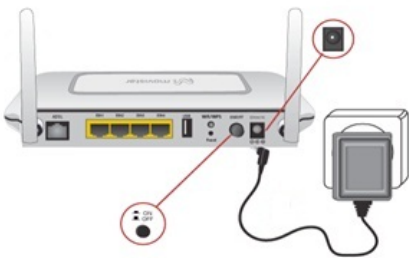
Figura 3.5 Conexión del Home Station ADSL a la red eléctrica
