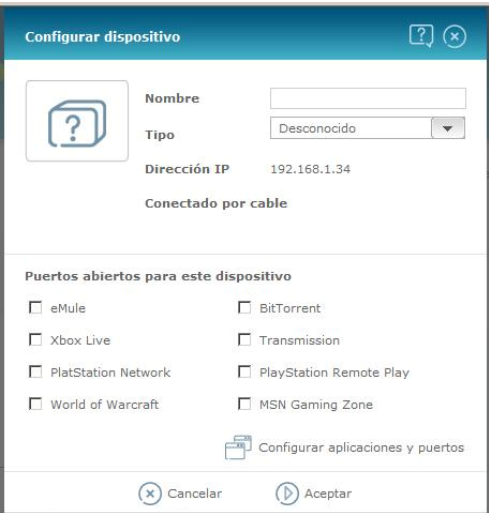
Figura 5.7 – Configurar dispositivo
