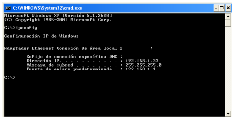
Figura 1.7 Resultado ‘ipconfig’
