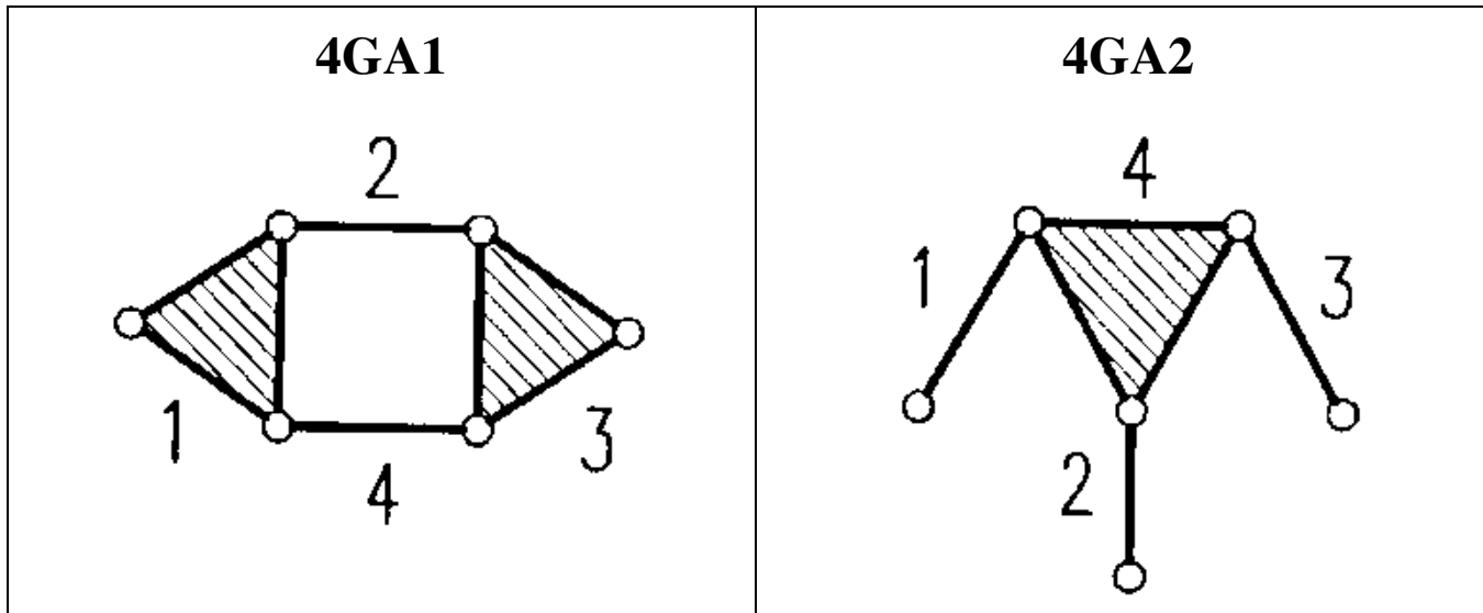
Grupos de Assur de cuatro eslabones
