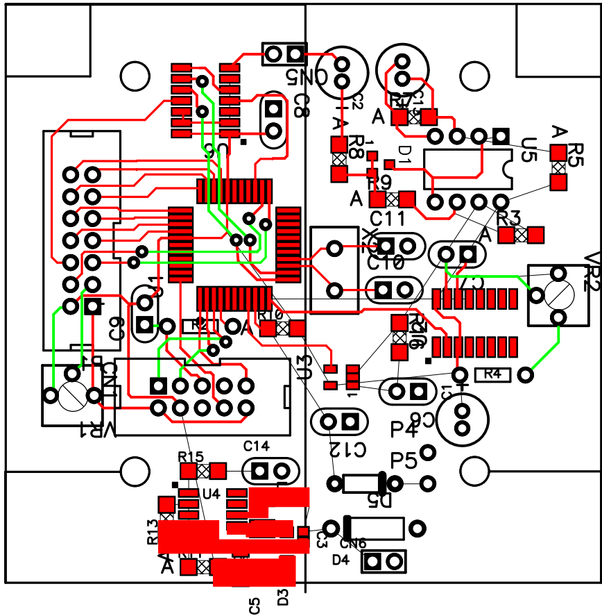
pactec pplx 9vb 2aa bottom pcb
