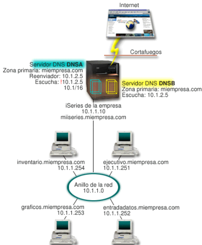
Figura 1. Dividir el DNS con un cortafuegos.
