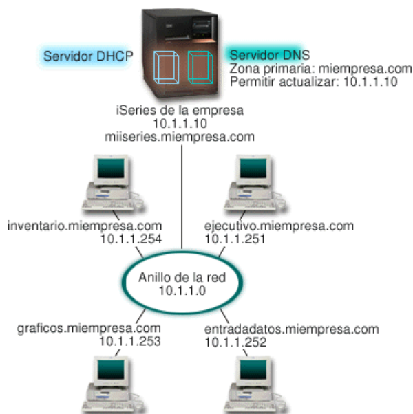
Figura 1. DNS y DHCP en el mismo servidor iSeries.
