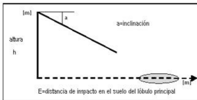
Figura 2. La distancia ( E ) de la superficie principal de incidencia del lóbulo en el suelo se obtiene por la fórmula: E = \tan(90-a) \times h , siendo a el ángulo de inclinación de la emisión de la antena respecto a la horizontal y h la altura a la que está instalada. (Adaptado de Eger et al., 2004).
