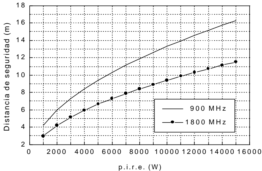
Figura 8. Distancia mínima de seguridad en función de la potencia radiada en el espacio libre
