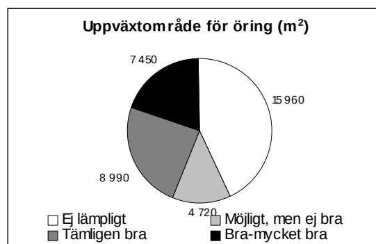
Figur 6. Diagram över fördelningen av lämpliga uppväxtområden för öring i Björkån. Data från inventeringar gjorda sommaren 2003.
