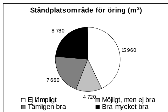
Figur 7. Diagram över fördelningen av lämpliga ståndplatsområden för öring i Björkån. Data från inventeringar gjorda sommaren 2003.
