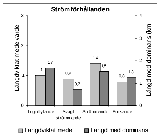
Figur 1. Diagram över rådande strömförhållanden i Björkån. Data från inventeringar gjorda sommaren 2003.
