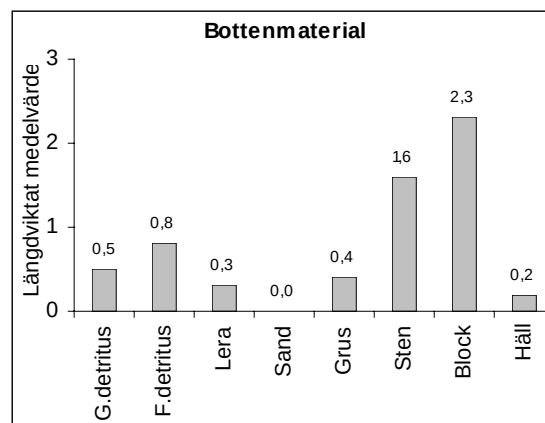
Figur 2. Diagram över bottensubstratens fördelning i Björkån. Data från inventeringar gjorda sommaren 2003.
