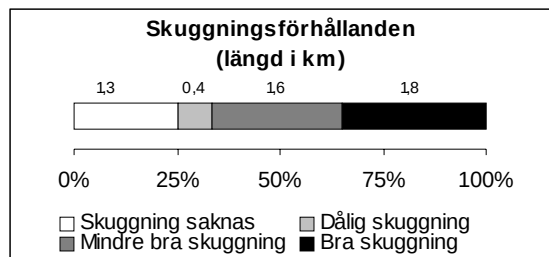
Figur 3. Diagram över hur Björkån skuggas av omgivande vegetation. Data från inventeringar gjorda sommaren 2003.
