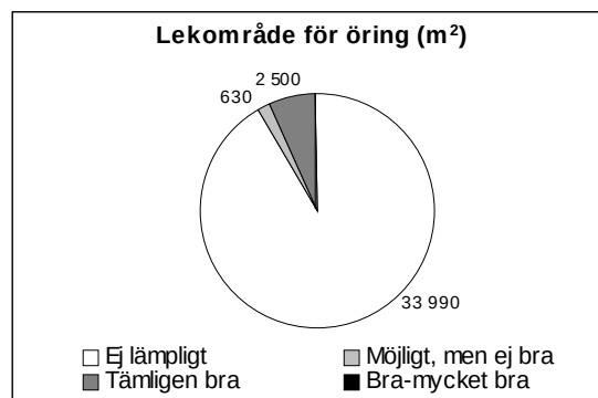
Figur 5. Diagram över fördelningen av lämpliga lekområden för öring i Björkån. Data från inventeringar gjorda sommaren 2003.
