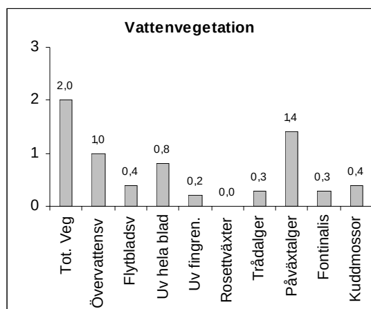
Figur 4. Diagram över vattenväxternas fördelning i Björkån. Data från inventeringar gjorda sommaren 2003.
