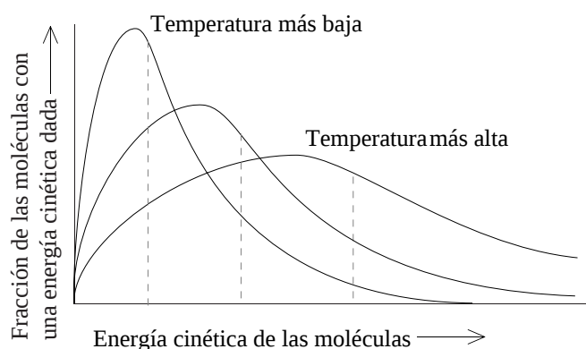
Figura 6.3. Distribución de las energías cinéticas de las moléculas de un gas, según la teoría cinético-molecular. Las energías cinéticas promedio se indican mediante líneas de trazos. Conforme aumenta la temperatura, la energía cinética promedio de las moléculas aumenta. A cualquier temperatura, una porción de las moléculas puede tener velocidades muy altas.
