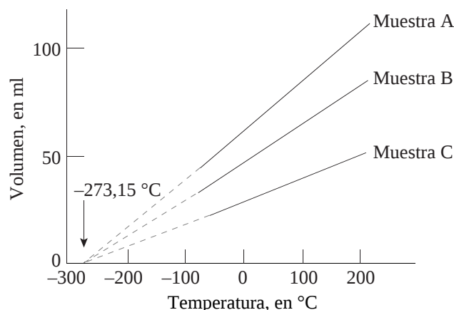
Figura 6.2. Ley de Charles. Representación gráfica del volumen frente a la temperatura para tres muestras gaseosas diferentes a presión constante. Cuando se extrapolan, las tres rectas cortan al eje de las temperaturas a -273\text{ °C} .
