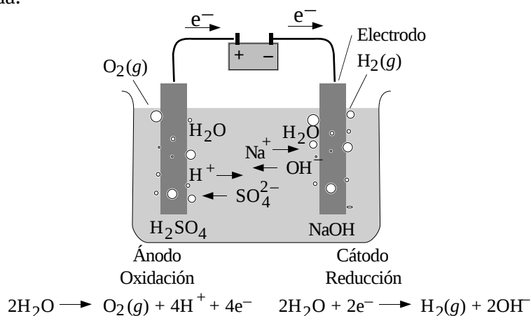
Figura 14.1. Electrólisis del agua. La adición de sulfato de sodio mejora la conductividad facilitando la electrólisis.
