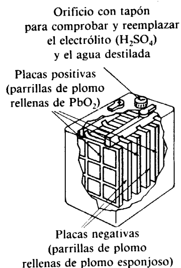
Figura 14.5. Acumulador de plomo
