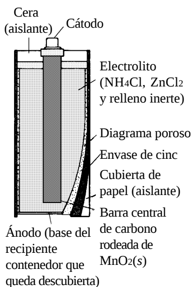
Figura 14.3. Pila seca
