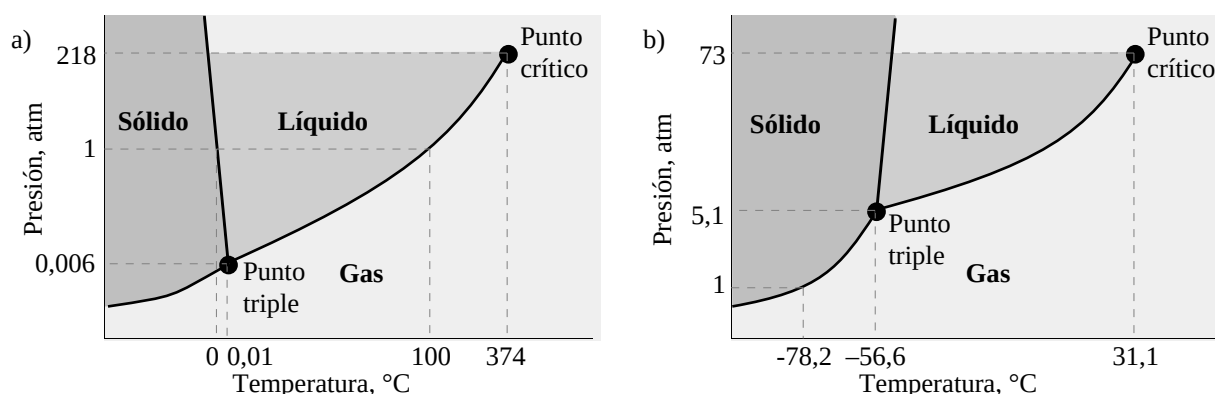
Figura 8.5. Diagrama de fases (no a escala) para a) el agua, b) el dióxido de carbono. Para el \text{CO}_2 , la temperatura de fusión aumenta con la presión. Esta es la situación general para casi todas las sustancias. La anomalía de la curva de fusión del agua se debe a que su volumen aumenta al congelar, y se puede explicar mediante el principio de Le Chatelier.
