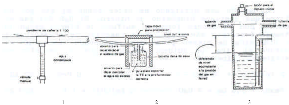
FIGURA 50: Tipos de drenaje: 1) Simple tipo "T"; 2) Automático subterráneo; 3) Automático tipo "sifón"
