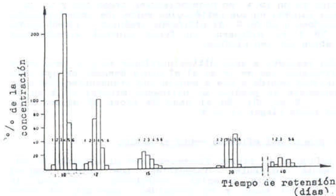
FIGURA 51: Reducción de las sustancias provocadoras de mal olor: 1 Fenol; 2 P-cresol; 3 Etil-fenol; 4 Indol; 5 Skatol; 6 Acido acético.
