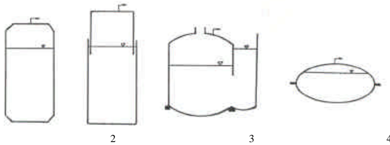
FIGURA 47: 1. Digestor cerrado; 2. Gasómetro flotante; 3. Campana fija; 4 Balón plástico
