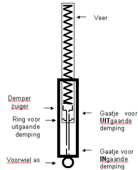
De opbouw van een voorvork
