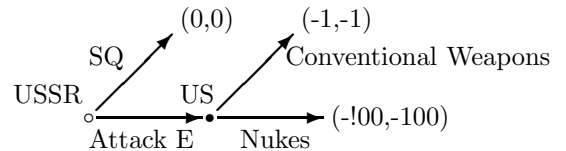
図 2: Extended Deterrence
