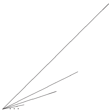
Figura 2.2: Dendrita F_\omega
