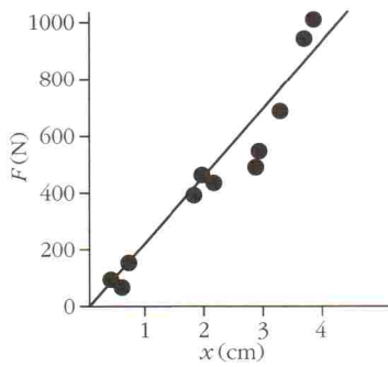
4. ábra. Erő-benyomódás grafikon
