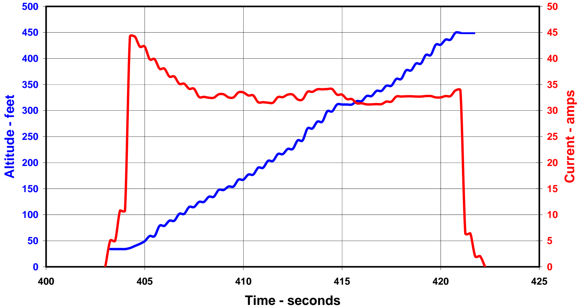
Graph 8 - Big Swift 45° climb (D).
