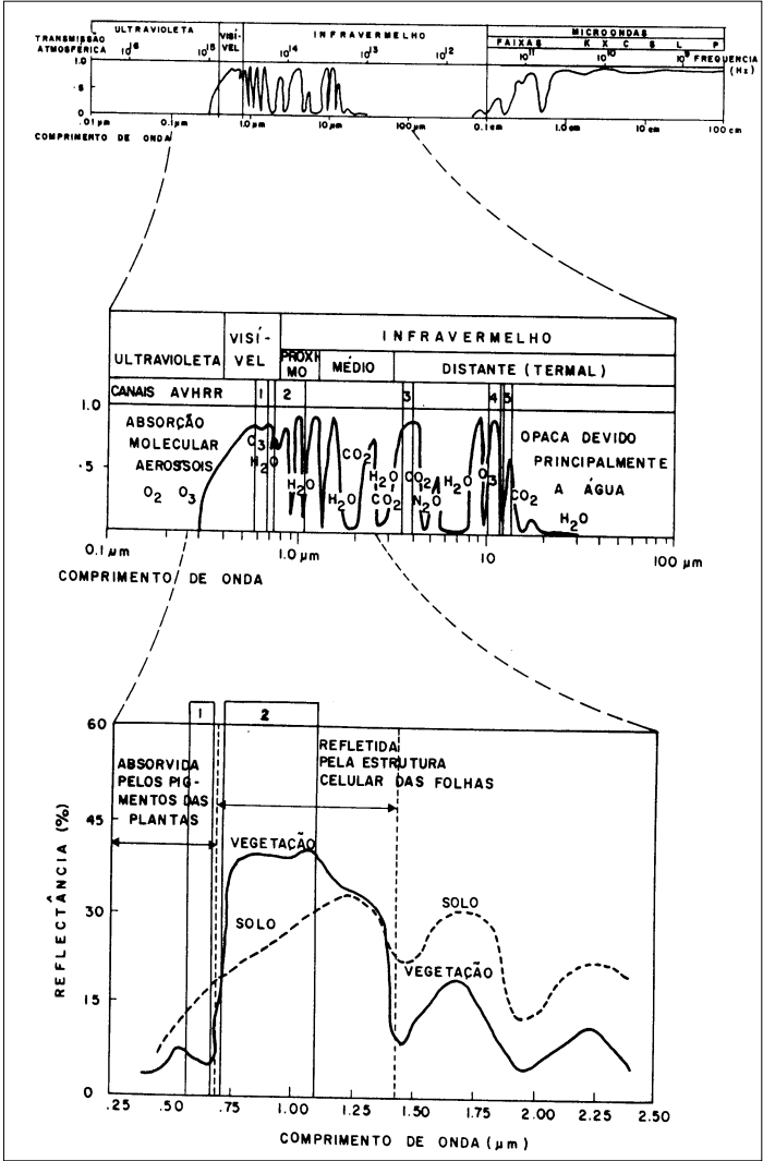
Figura 1: Espectro eletromagnético mostrando a janela atmosférica, posição das bandas do AVHRR, e as curvas espectrais de vegetação e de solo.
