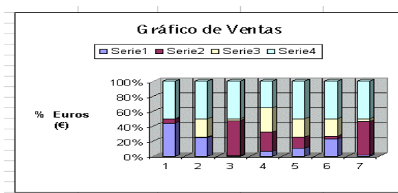
Figura 49. Gráfico.
