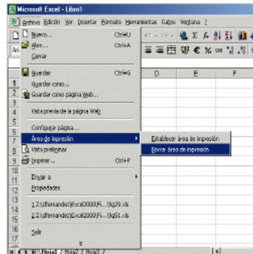
Figura 4. Menú Archivo.
