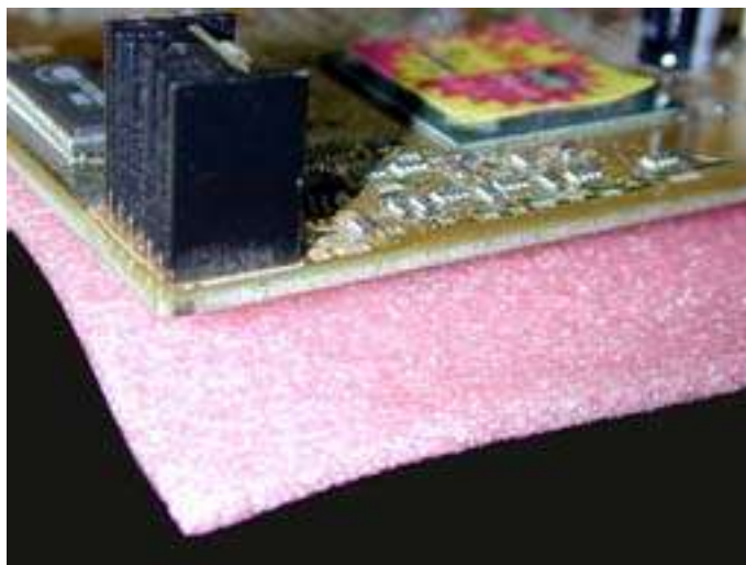
Figura 7: Espuma antiestática não deve ser instalada embaixo da placa-mãe!
