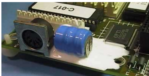
Figura 17b - Protegendo a placa mãe com cola plástica.
