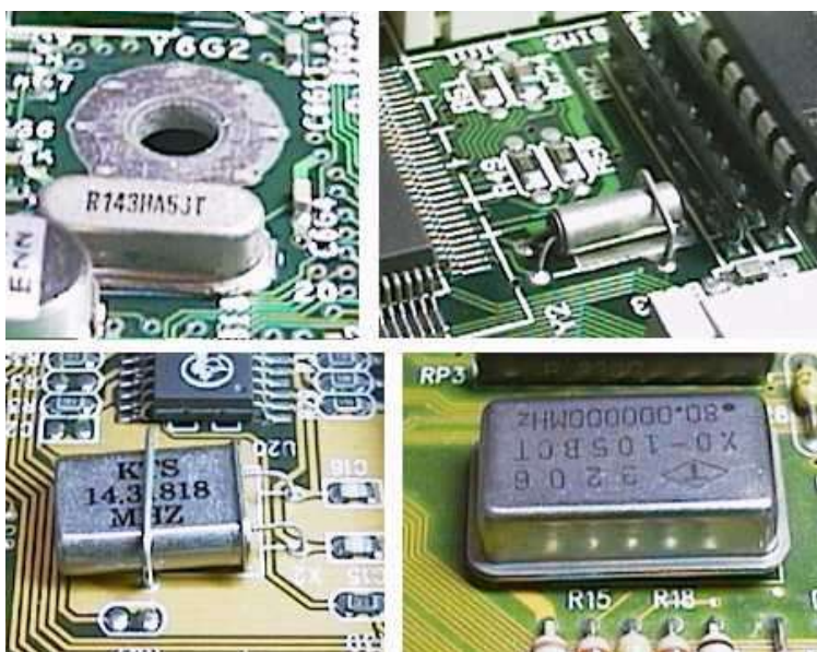
Figura 14 - Cristais – podem apresentar diversos formatos, mas seu encapsulamento é sempre metálico.
