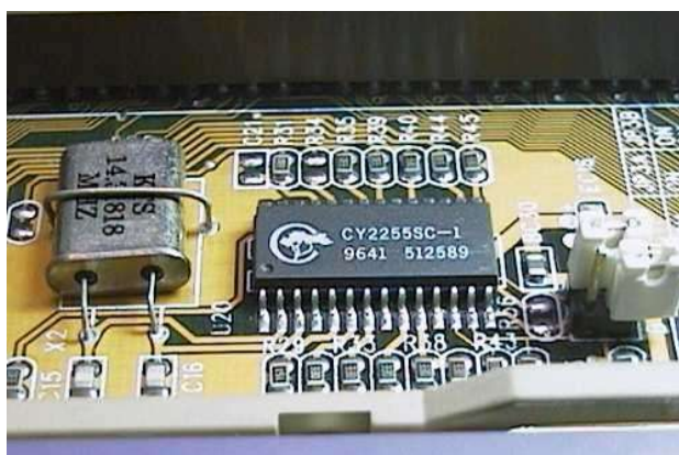
Figura 15 - Um chip sintetizador de clock. Observe o cristal 14.31818 MHz ao seu lado, bem como os jumpers para seccionamento do clock externo do processador.
