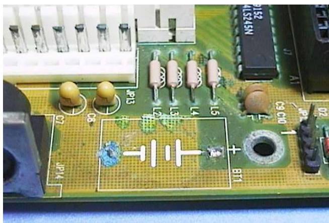
Figura 17a - Uma bateria com vazamento. Observe o ataque que o ácido fez na placa.
