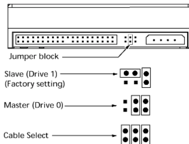
Figura 3.16 Jumpers de um ZIP Drive IDE.
