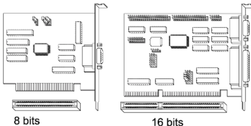
Figura 1.10 - Placas de expansão e slots ISA de 8 e de 16 bits.
