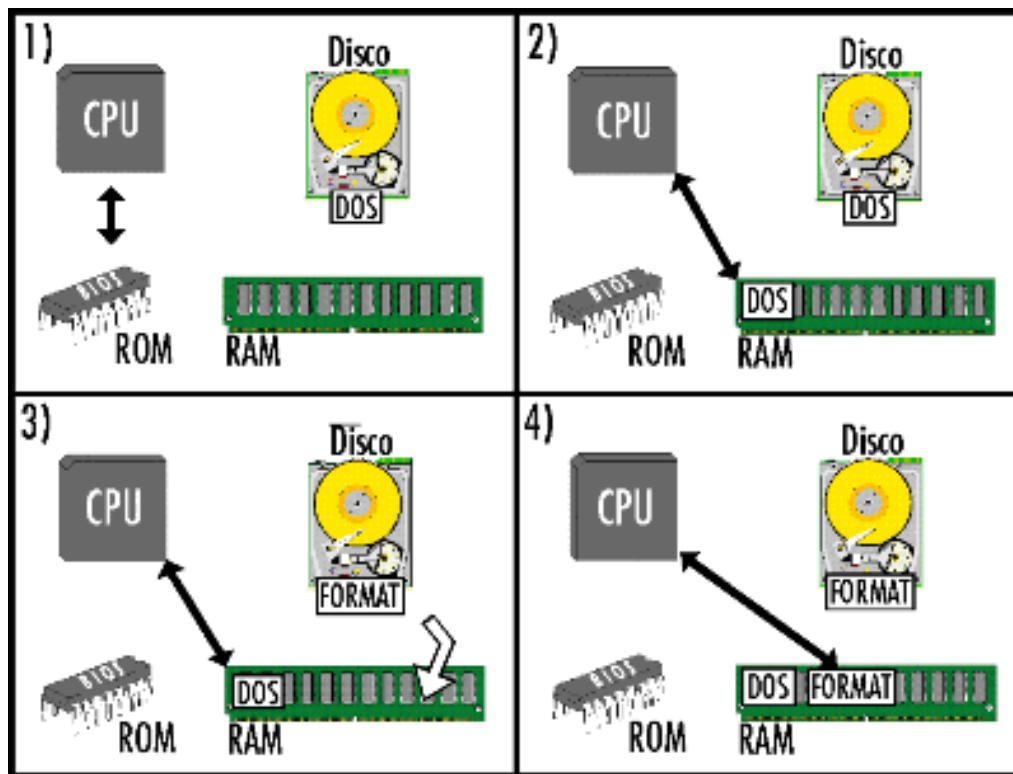
Figura 25 - BOOT e carga de um programa
