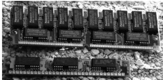
Figura 13 - Módulos de memória
