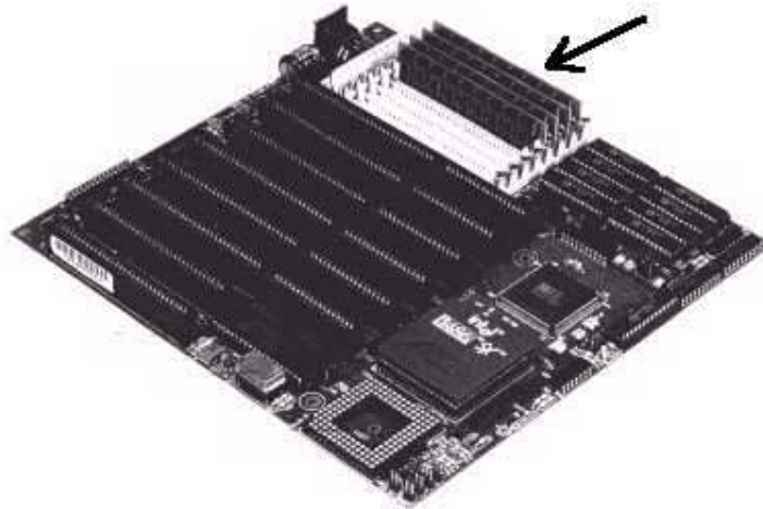
Figura 17 - Placa de CPU e suas memórias
