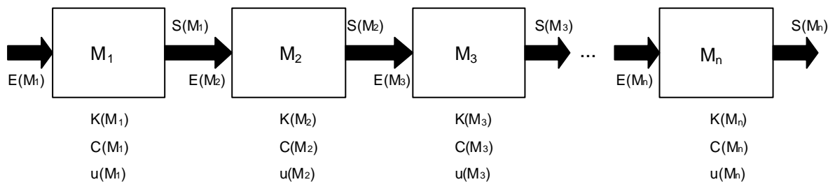
Figura 10.1 - Propagação de incertezas entre módulos interligados de um Sistema de Medição
