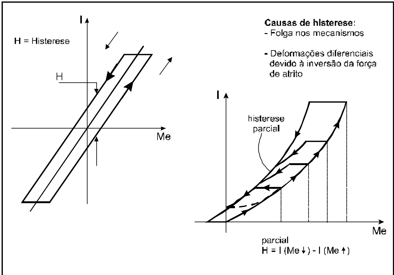
Figura 3.8 - Histerese
