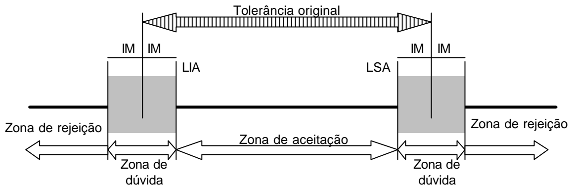
Figura 7.1 – Zonas de aceitação, de rejeição e de dúvida ao verificar-se uma tolerância.
