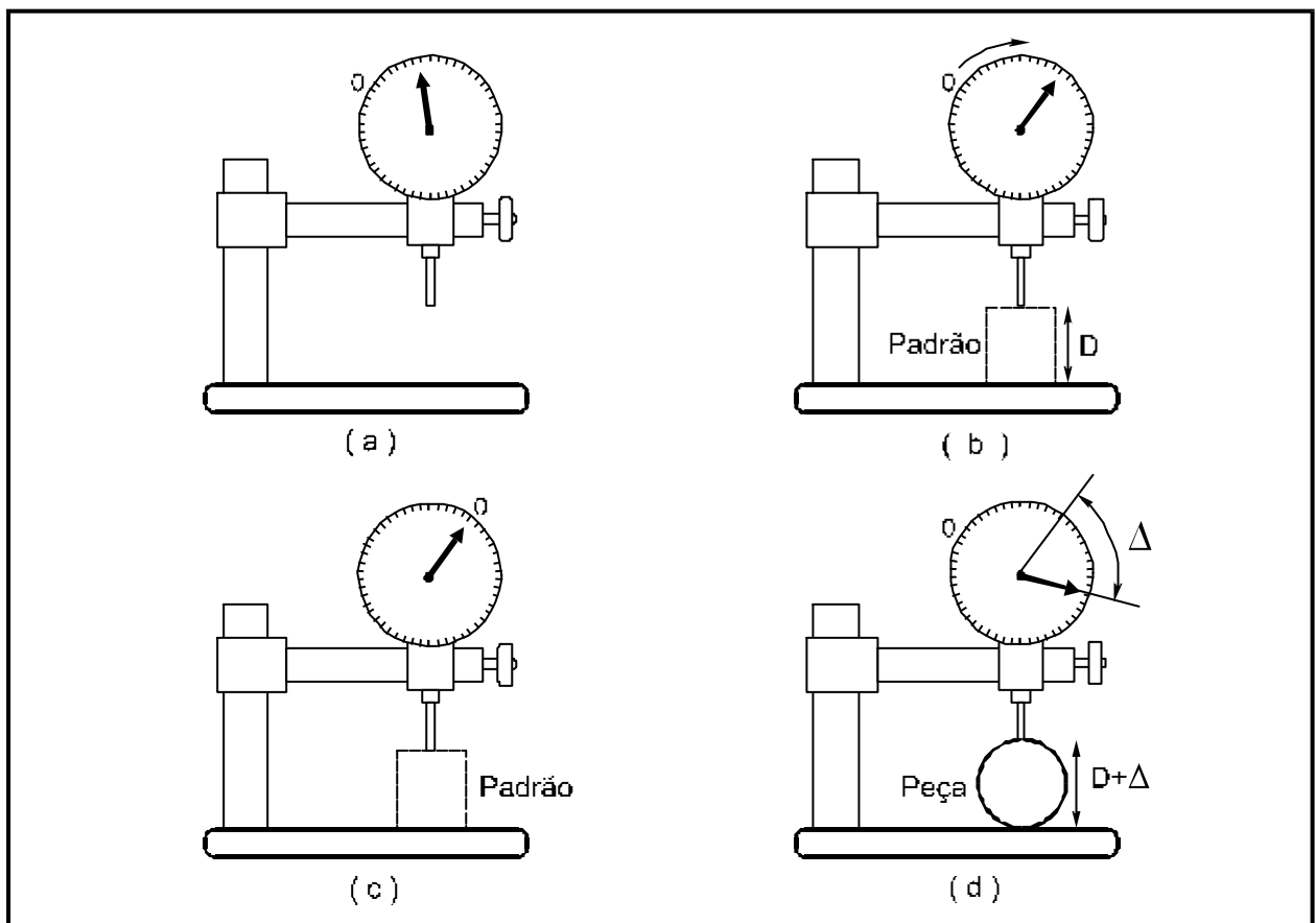
Figura 2.4 - Medição Diferencial
