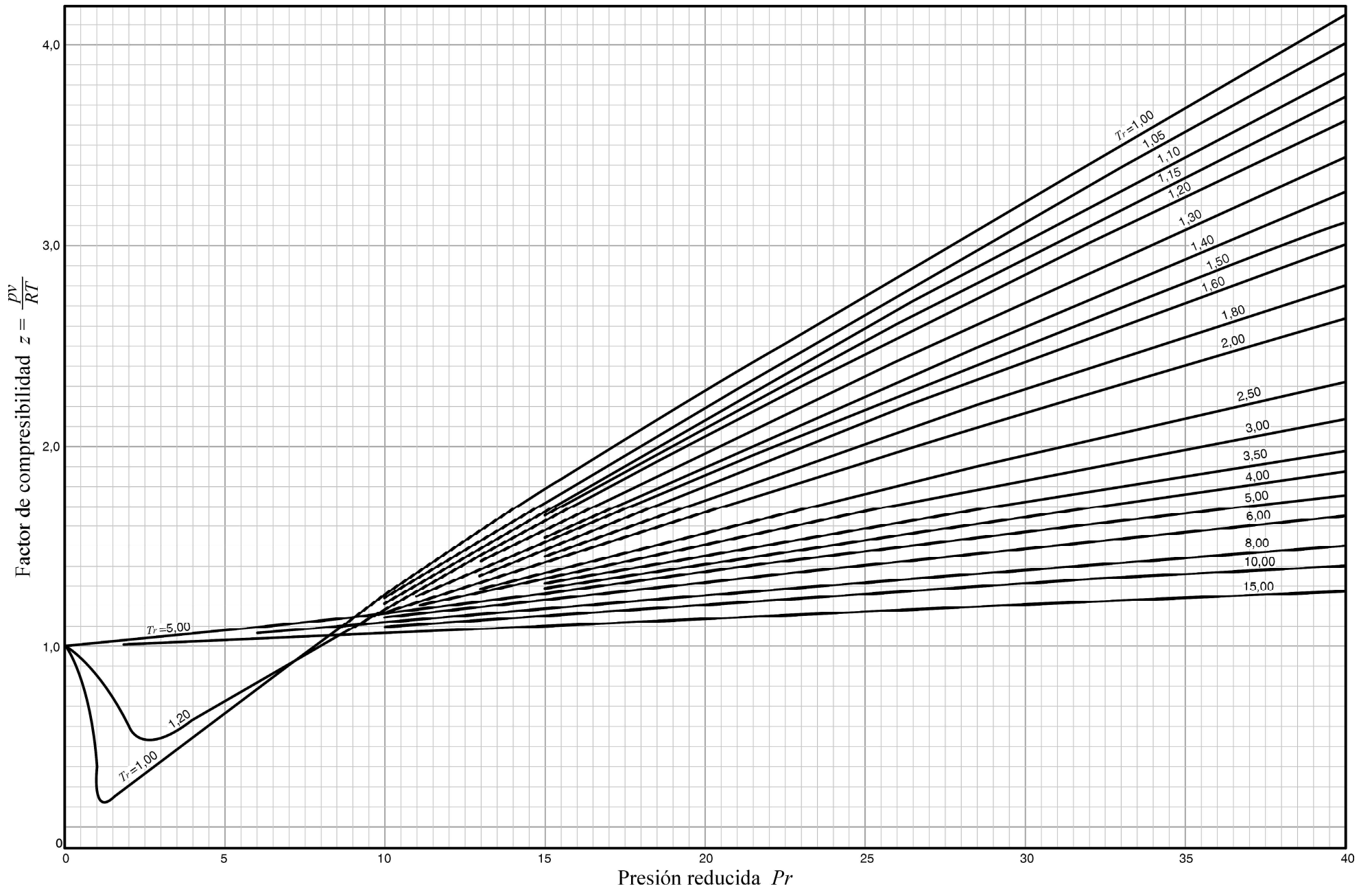
Diagrama de compresibilidad generalizado de Nelson-Obert (presiones altas).
