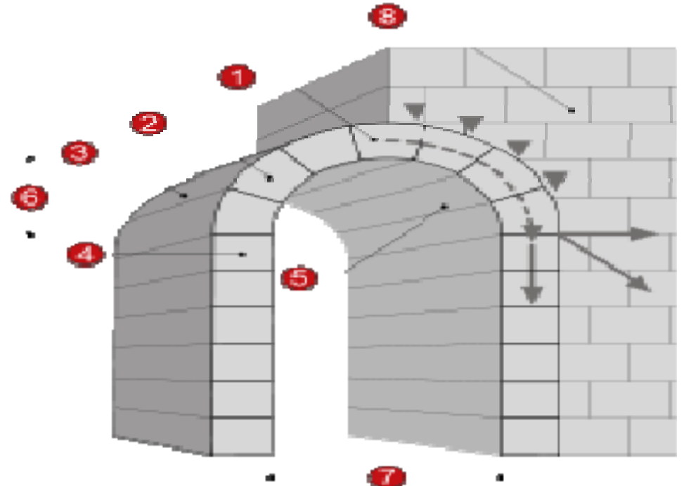
Esquema de un Arco, "Romano" o de "Medio Punto" y la Bóveda, Cilíndrica o "De Cañón", generada, por el Arco:
