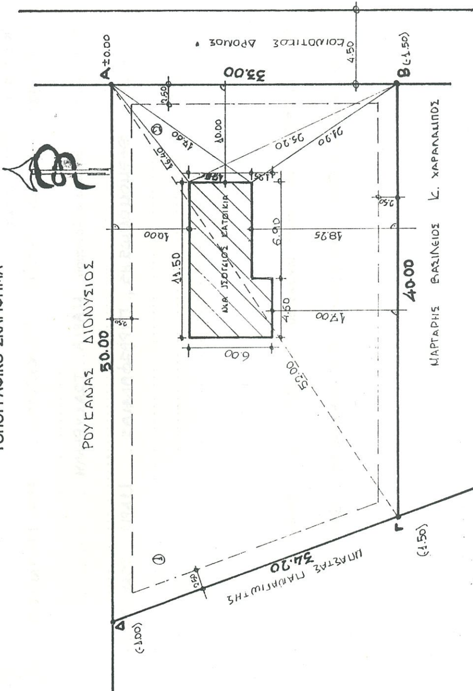
ΤΟΠΟΓΡΑΦΙΚΟ ΣΚΑΡΙΦΗΜΑ
