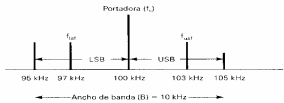
Figura 3-3 Espectro de salida para el ejemplo 3-1.
