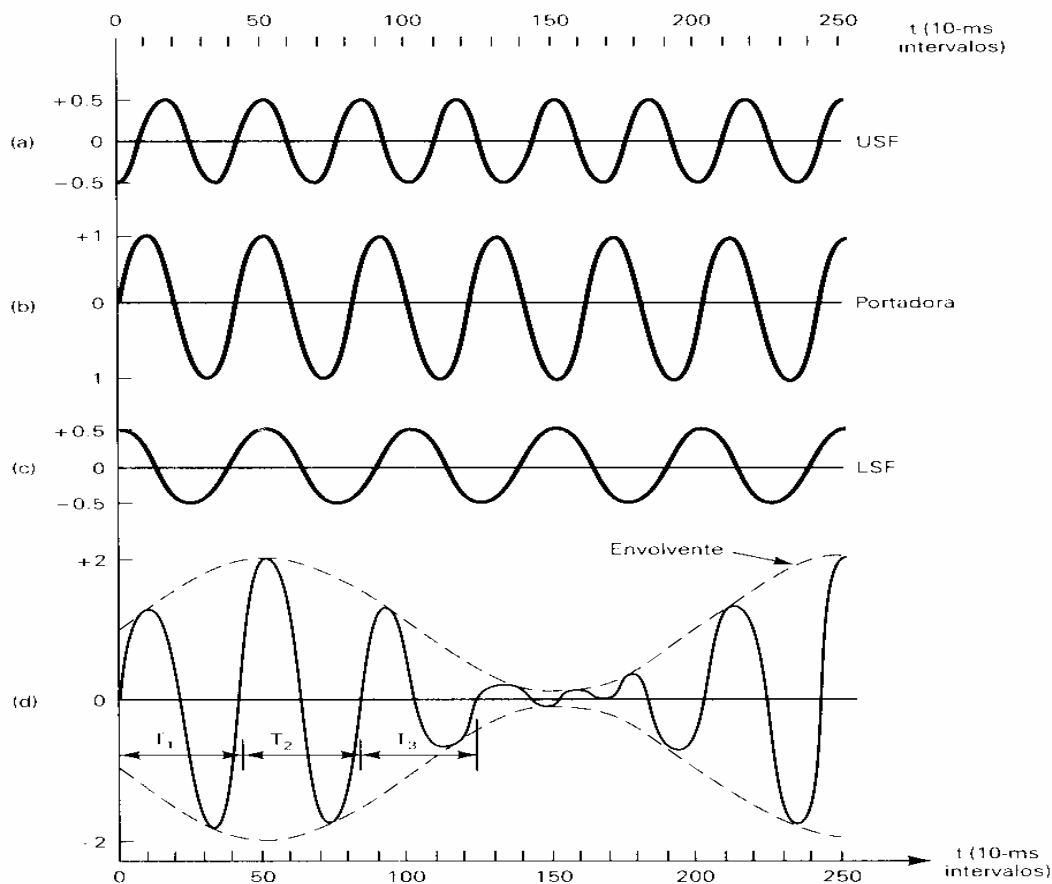
Figura 3-9 Generación de una envolvente de AM DSBFC mostrada en el dominio de tiempo: (a) -1/2\cos 2\pi 30t ; (b) \text{sen} 2\pi 25t ; (c) +1/2\cos \pi 20t ; (d) suma de (a), (b) y (c).
