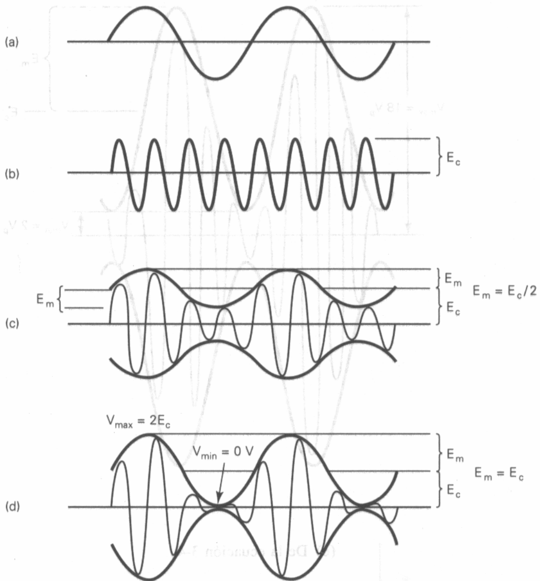
Figura 3-6 Porcentaje de modulación de una envolvente de AM DSBFC (a) señal modulante; (b) portadora no modulada; (c) onda modulada 50%; (d) onda modulada 100%.
