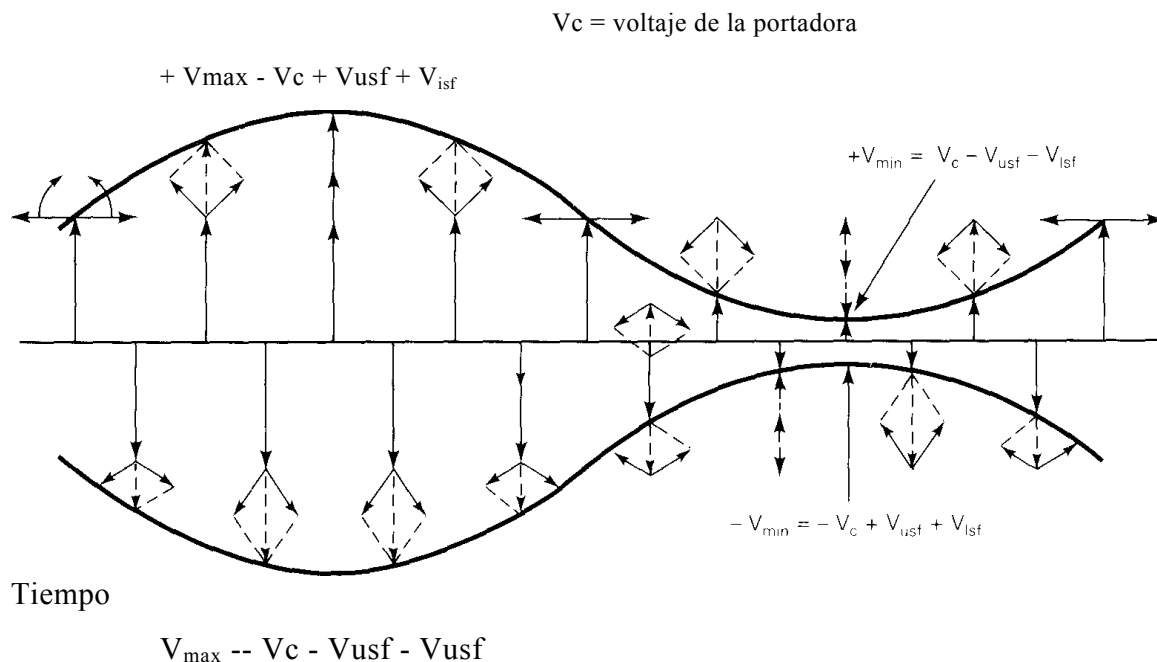
Figura 3-4 La adición fasorial en una envolvente de AM DS13FC: (a) adición fasorial de la portadora y las frecuencias laterales superior e inferior; (b) adición fasorial produciendo una envolvente de AM.
