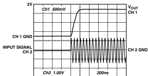
TPC 16. V_{OUT} Rise Time
