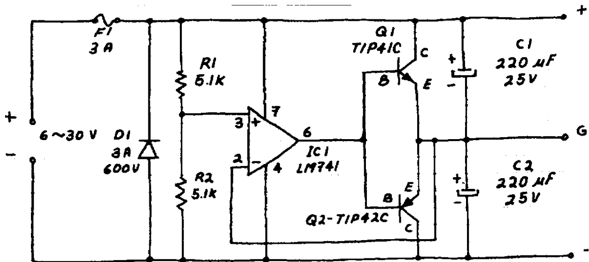
Convertidor de fuente simple a dual
