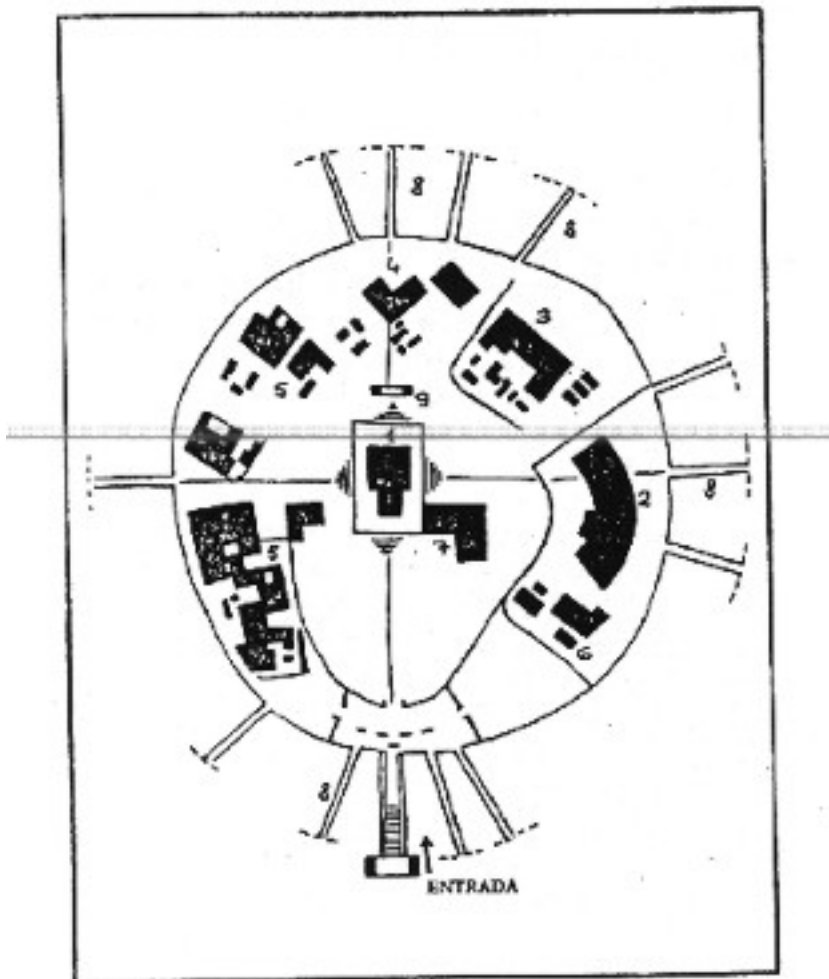
Grande plano da Baixa Akakor. 1 — templo; 2 — palácio; 3 — sacerdotes; 4 — arsenal; 5 — povo; 6 — palácio dos guardas; 7 — sala do trono; 8 — corredores de comunicação; 9 — portão dos Deuses
