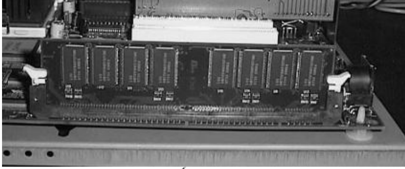
র্যাম — মাদারবোর্ডে লাগানো অবস্থায়
